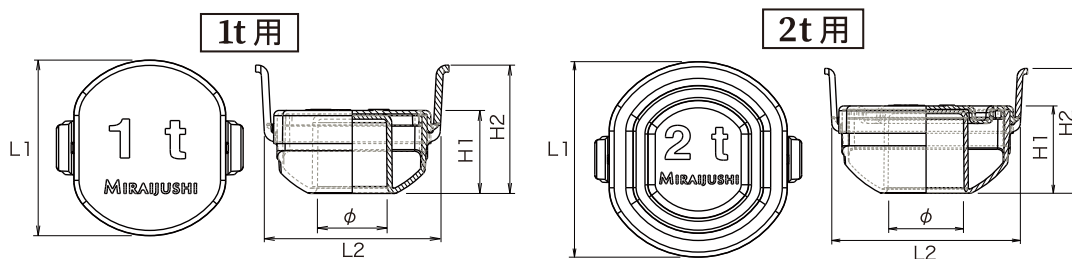
■アンカーキャップ 仕様
