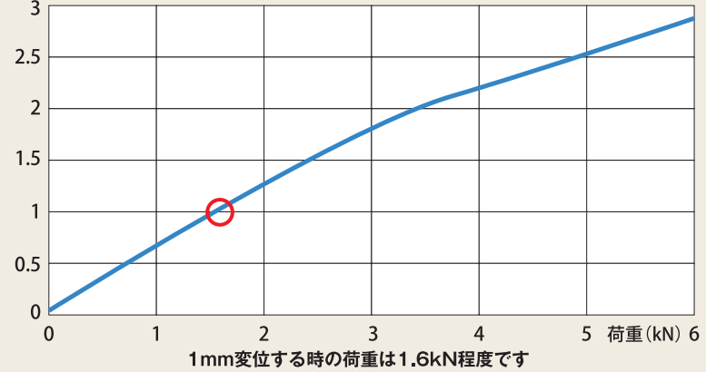
変位(mm) パネルパット60φS 4点使用時 圧縮荷重—変位曲線
